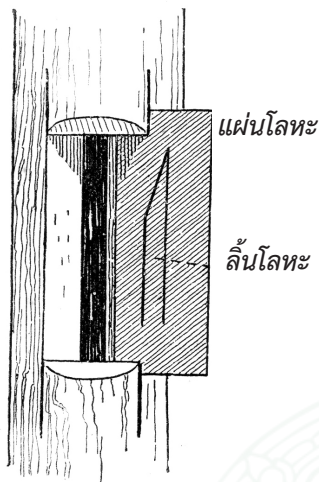
ท่อปีของแคน
