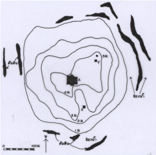
ผังแสดงหลุมขุดค้นที่แหล่งโบราณคดีบ้านโนนวัดและคันน้ำ - คันดินทรงกลมล้อมรอบแหล่งโบราณคดี
