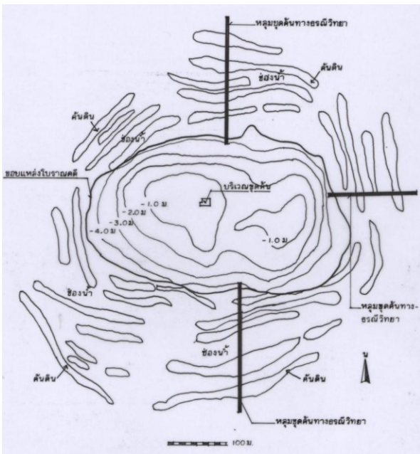
ผังแสดงบริเวณที่ขุดค้นแหล่งโบราณคดีเนินอุโลก และคูน้ำ-คันดินทรงกลมล้อมรอบแหล่งโบราณคดี
