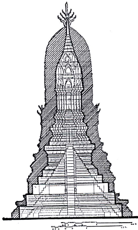
ลายเส้นที่ 55 แสดงการสร้างพระปรางค์สมัยอยุธยาครอบเจดีย์ยอดดอกบัวตูม
