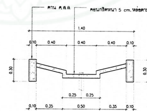
แบบขยาย D-5
