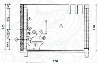
รูปด้านภายใน 3 ๑:๕๒ มาตราส่วน 1:50
