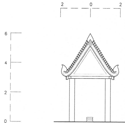
รูปด้าน 1 (ทิศตะวันออก) SCALE 1:75
