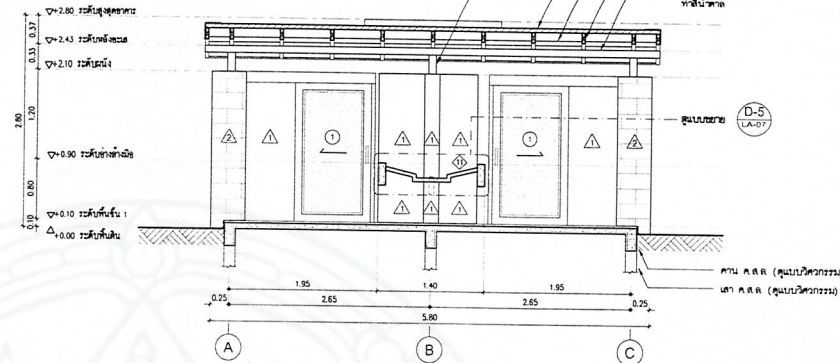
รูปตัด 4
