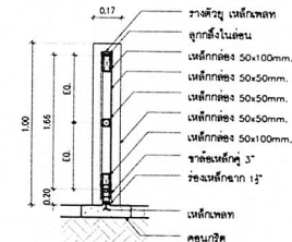
แบบขยายประตูเลื่อน ๑/๒ มัดรวม 1:25
