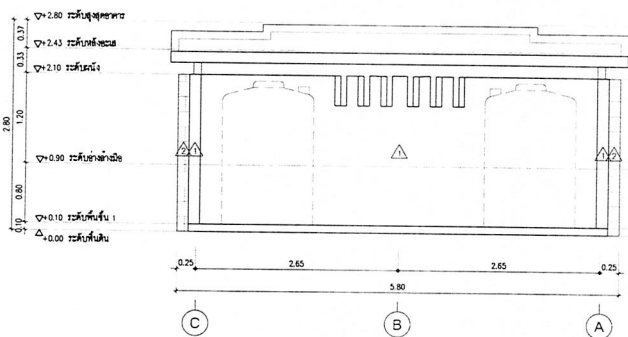
รูปตัด 3
