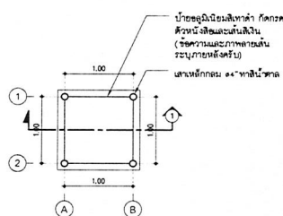
แปลน INFO. ๑:๕๒ มาตราส่วน 1:50
