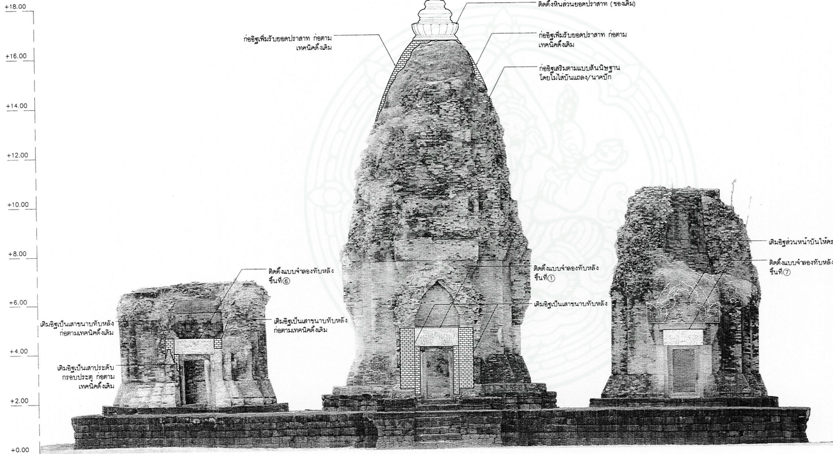
รูปด้าน 1 (ทิศตะวันออก)
