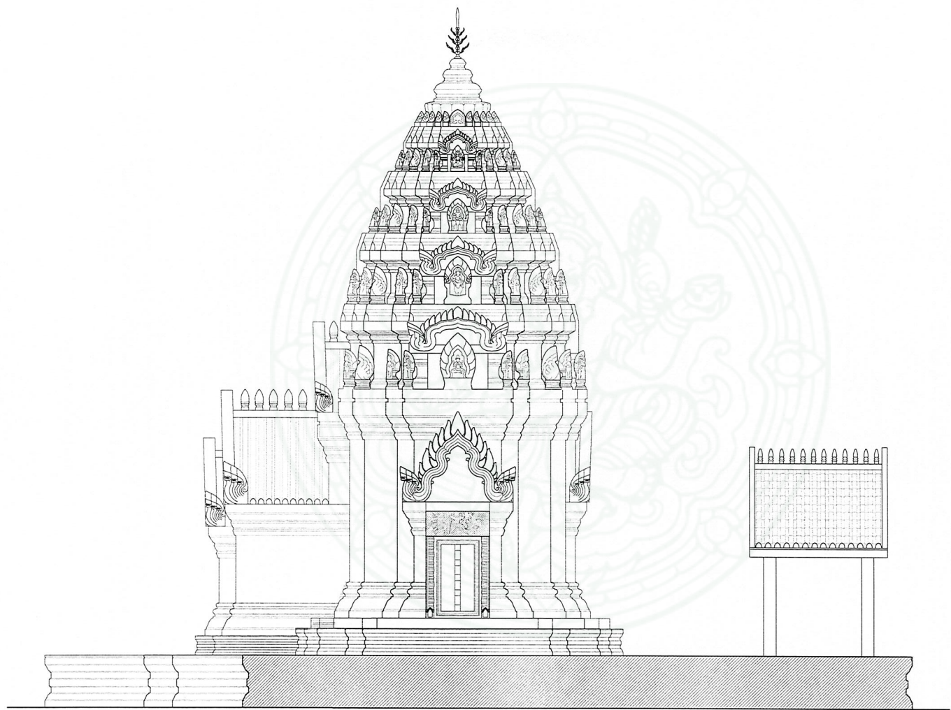
รูปด้าน 5 (ทิศเหนือ) ของปราสาทองค์กลาง 0 1 3 6 10
