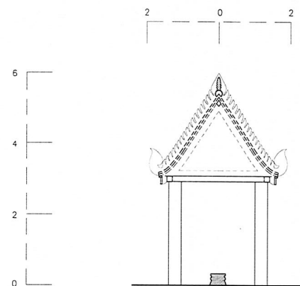
รูปตัด 1
