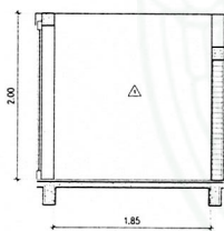
รูปด้านภายใน 4 ๑:๕๒ มาตราส่วน 1:50
