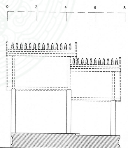
รูปตัด 2 SCALE 1:75
