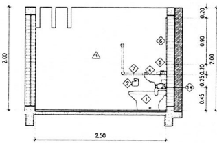
รูปด้านภายใน 3 ๑:๕๒ มาตราส่วน 1:50
