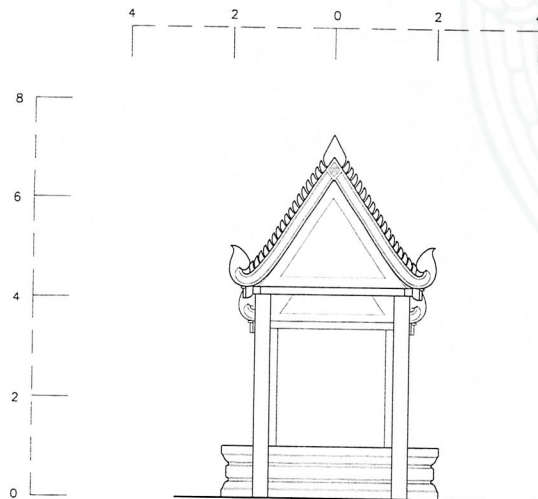
รูปด้าน 3 (ทิศตะวันตก) SCALE 1:75
