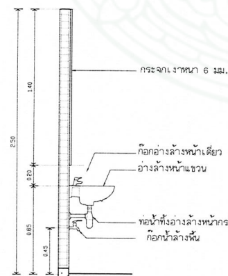
อ่างล้างหน้าติดผนัง LAV
