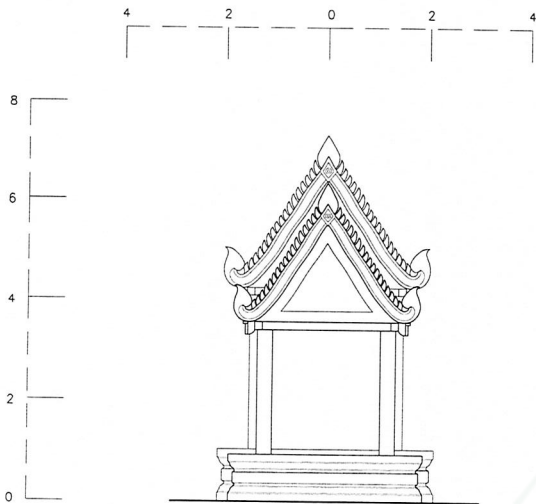
รูปด้าน 1 (ทิศตะวันออก) SCALE 1:75
