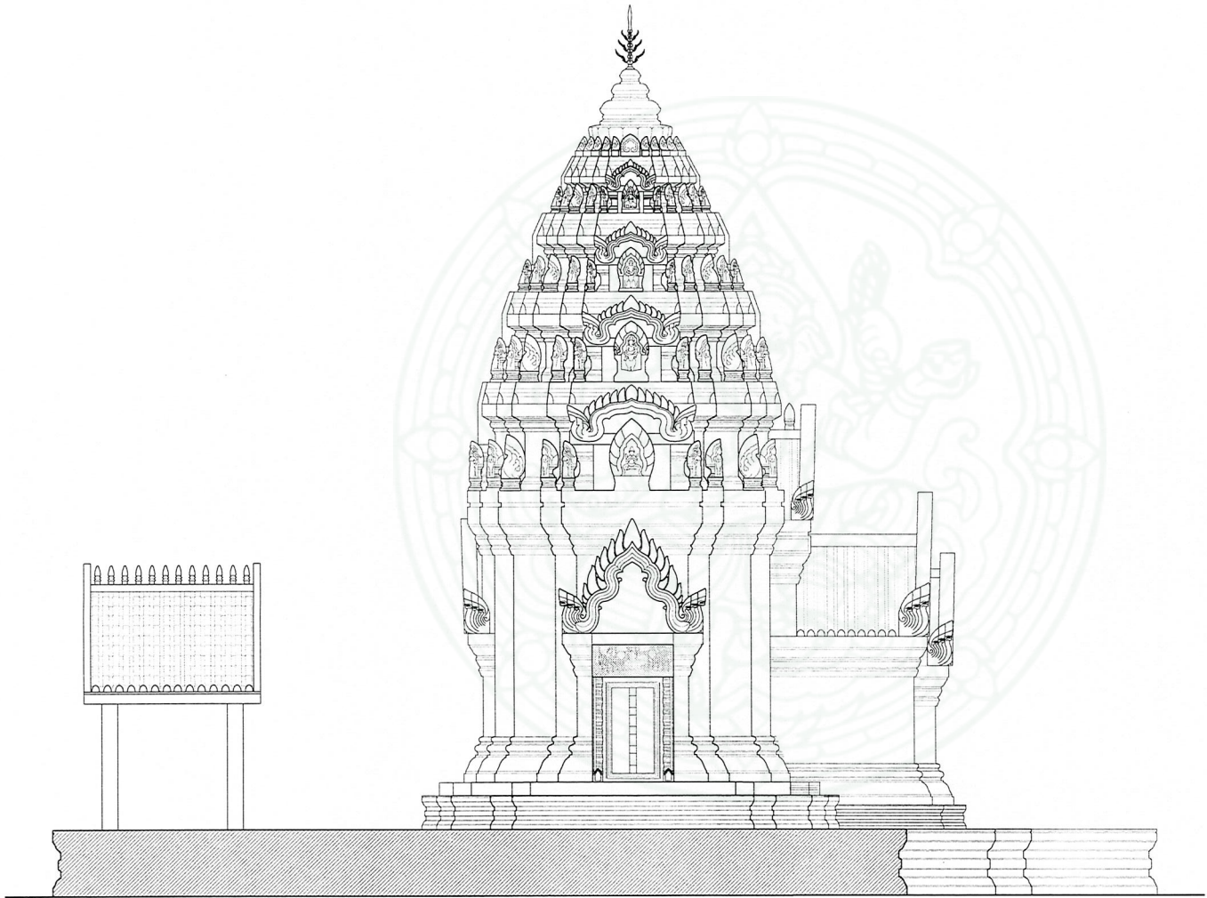
รูปตําน 6 (ทิศใต้) ของปราสาทองค์กลาง
