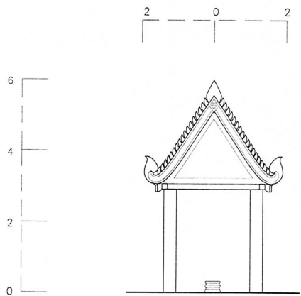
รูปด้าน 3 (ทิศตะวันตก) SCALE 1:75
