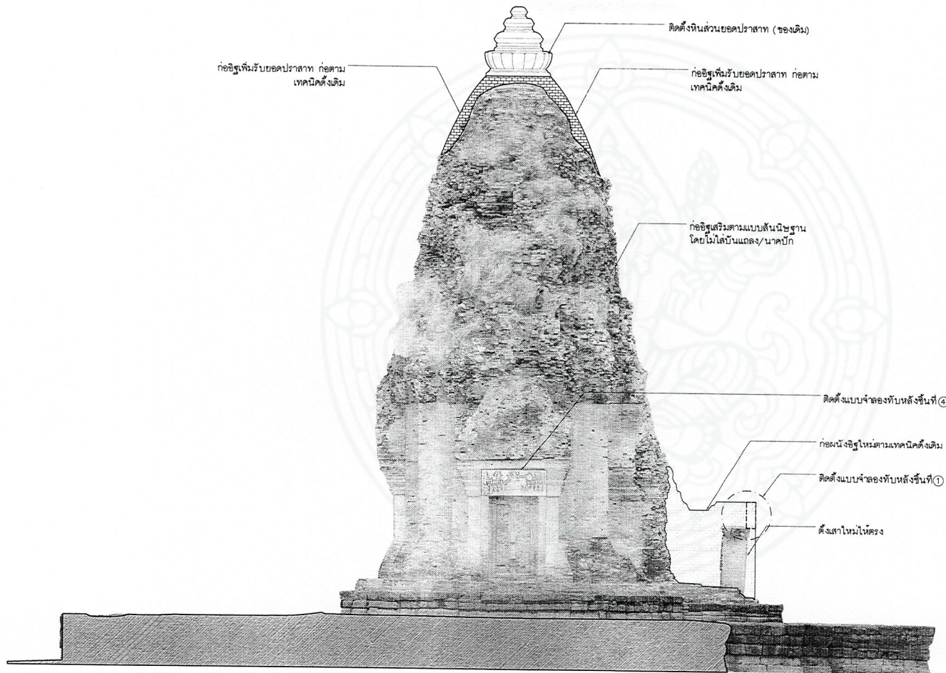
รูปด้าน 4 (ทิศใต้)
