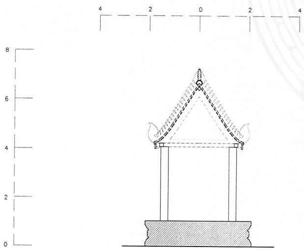
รูปตัด 1 SCALE 1:75
