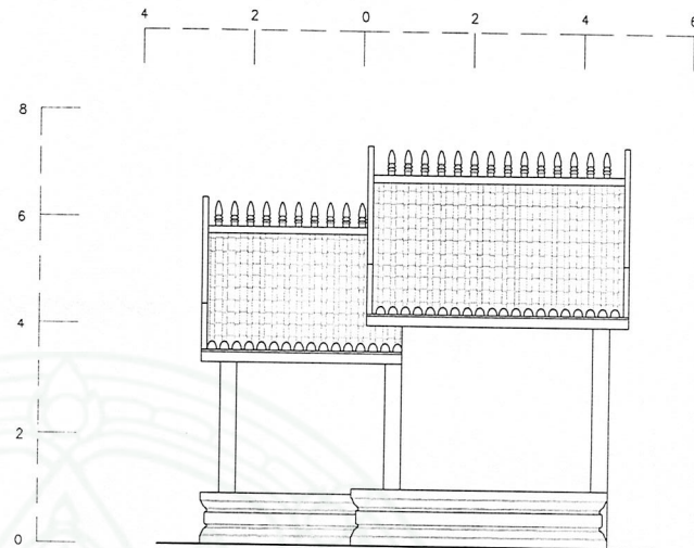
รูปด้าน 2 (ทิศเหนือ) SCALE 1:75
