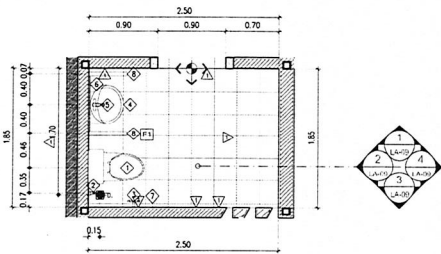
แปลนห้องชาย ๑:๕๒ มาตราส่วน 1:50
