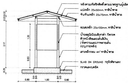
รูปด้าน 1 ๑:๕๒ มาตราส่วน 1:50
