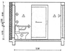
รูปด้านภายใน 1 ๑:๕๒ มาตราส่วน 1:50
