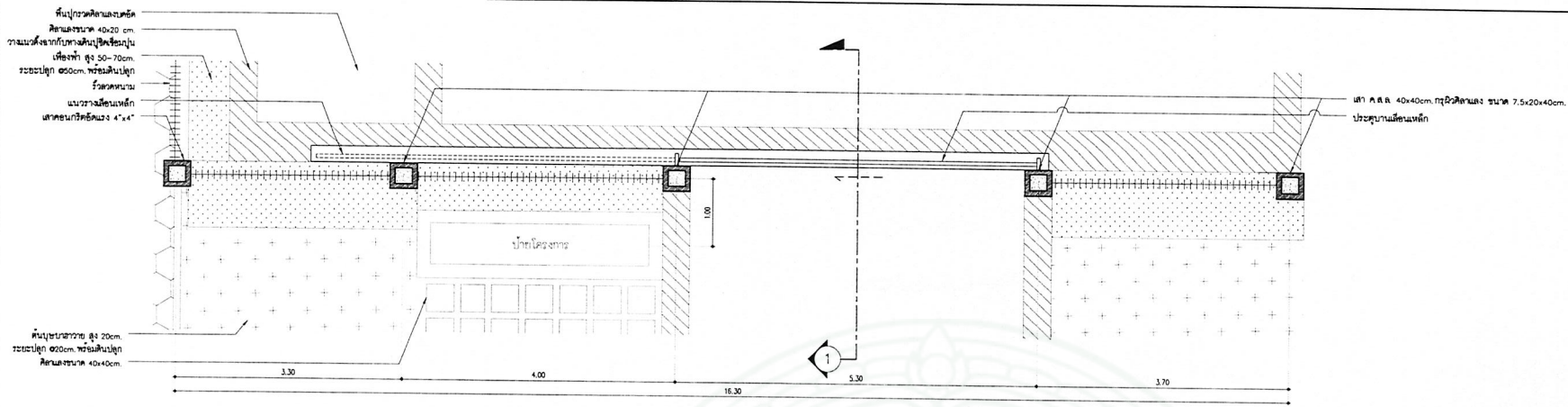
แปลนประตูทางเข้า ๑/๒ มัดรวม 1:50
