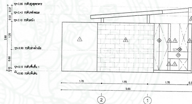
รูปตัด 5
