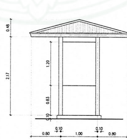
รูปด้าน 1 ๑:๕๒ มาตราส่วน 1:50
