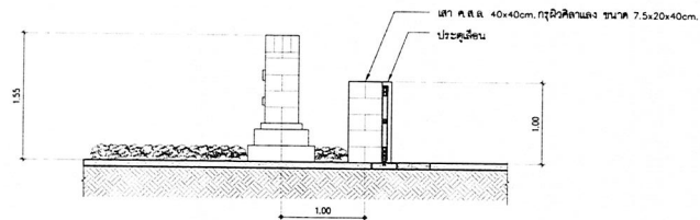
รูปตัด 1 ๑/๒ มัดรวม 1:50
