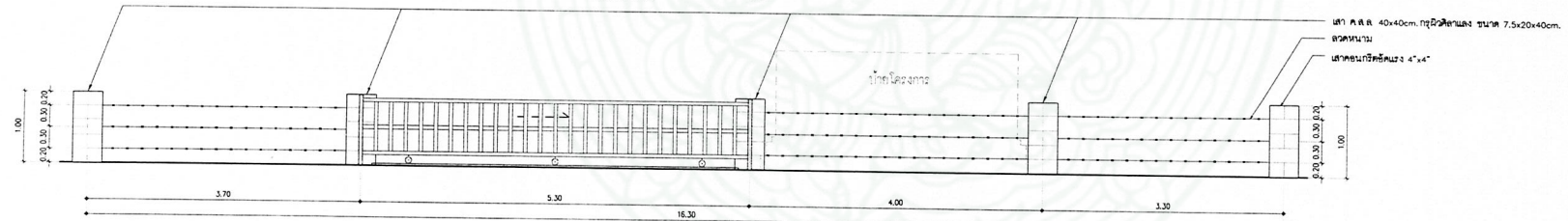
รูปด้าน 2 ๑/๒ มัดรวม 1:50
