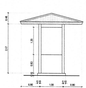
รูปด้าน 2 ๑:๕๒ มาตราส่วน 1:50
