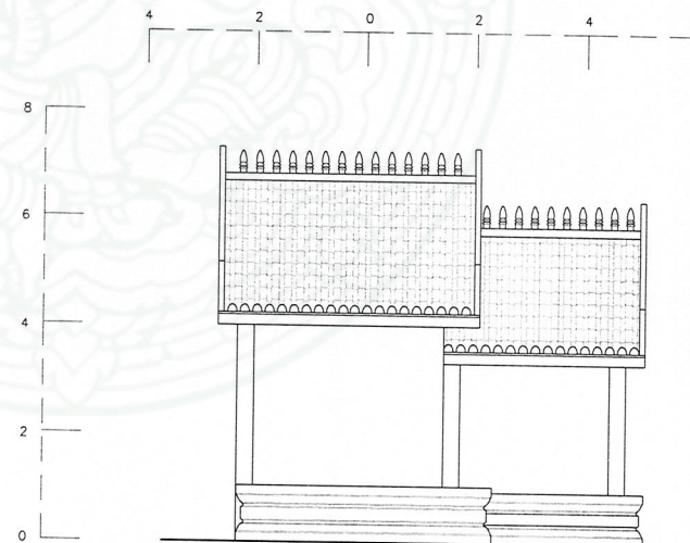
รูปด้าน 4 (ทิศใต้) SCALE 1:75
