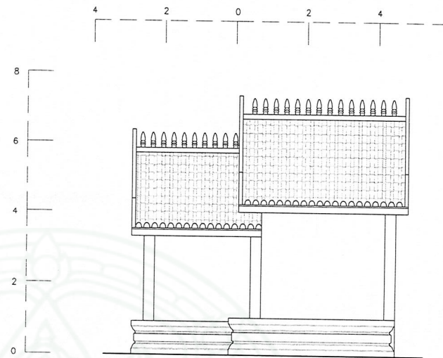
รูปด้าน 2 (ทิศเหนือ) SCALE 1:75
