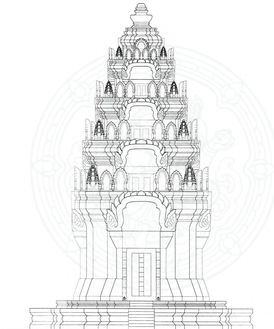
รูปด้าน 3 (ทิศตะวันตก): แบบที่ 2
