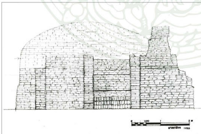
ภาพลายเส้นแสดงรูปเตาหลังเต่าที่เกาะเกร็ด (ด้านข้าง)
