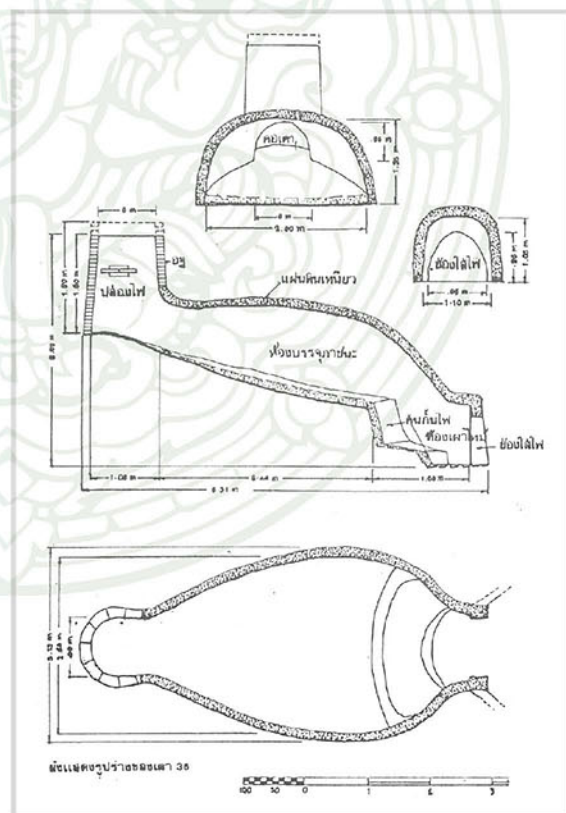
เตาแบบประทุนจากแหล่งเตาบ้านเกาะน้อย ต.หนองอ้อ อ.ศรีสัชนาลัย จ.สุโขทัย
